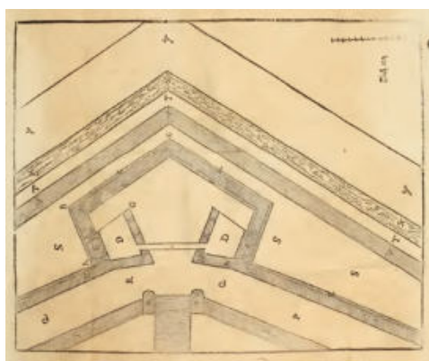
Fig. 8- “Come si debbiano fare i baluardi” (Lanteri, 1559, I, pp. 7-10)
