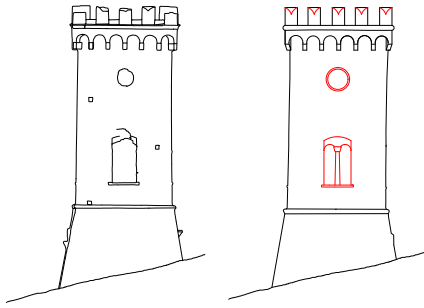
Fig. 12- Ipotesi ricostruttiva, sulla base della documentazione fotografica, di alcuni elementi architettonici sul prospetto Sud-Est (dx) a confronto con la condizione rilevata (sx) (elaborazione grafica degli autori)
