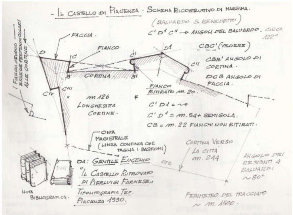
Fig. 1- Schema di costruzione geometrica della Cittadella pentagonale di Piacenza (elaborazione grafica di Francesco Broglio, 2022)
