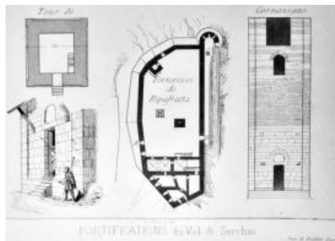
Fig. 3 - De Fleury, 1873, Tav. XLIX, Plan général - Coupe - Plan détaillé - Torre di Cornazzano
