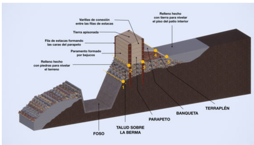
Fig. 7- Sección tridimensional del reducto de San Fernando (elaboración propia a partir del plano original, usando Revit 2022)
