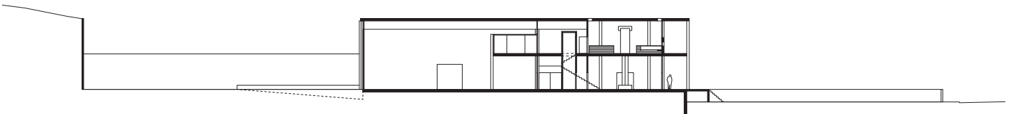
Sección transversal. Cross Section
