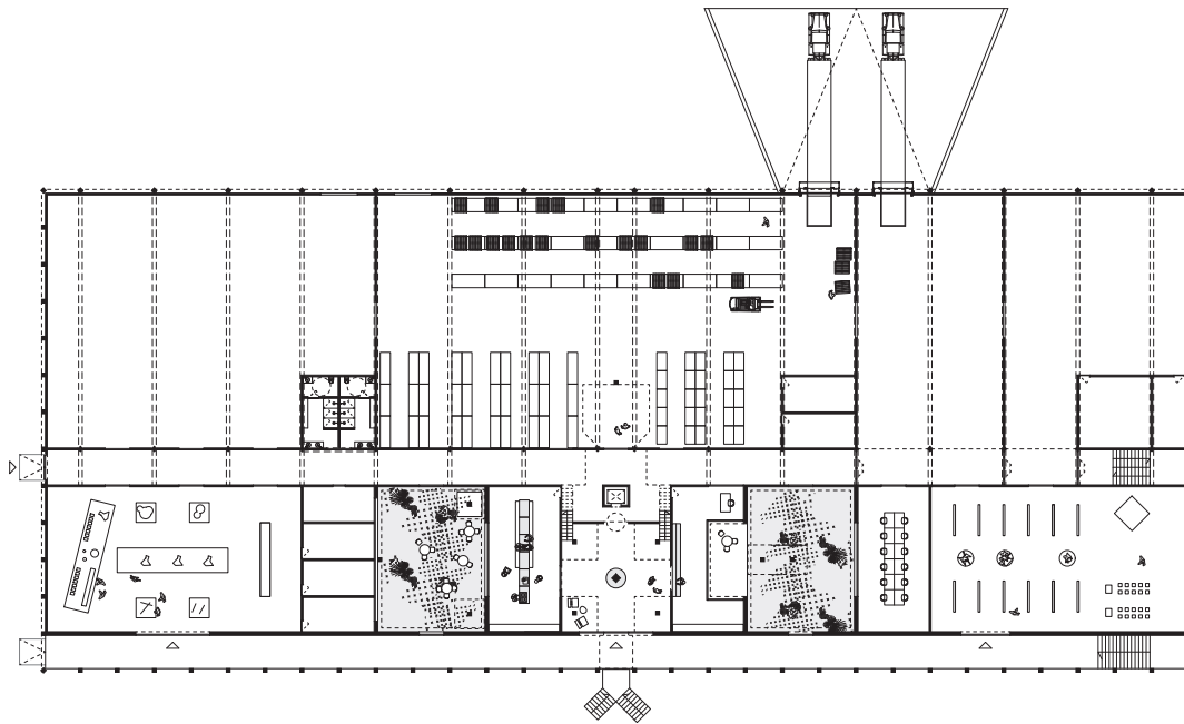
Planta baja. Ground Floor Plan
