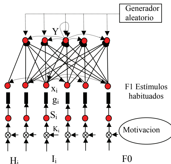
Figura 3. Arquitectura neuronal.
