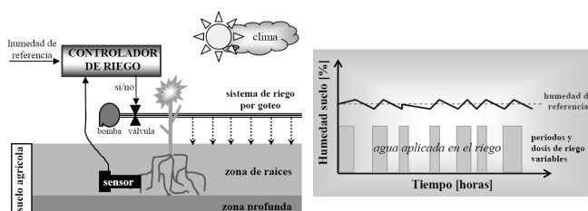
Figura 2. Control de riego basado en la humedad del suelo (lazo cerrado). Dosis de riego variables en periodos irregulares.
