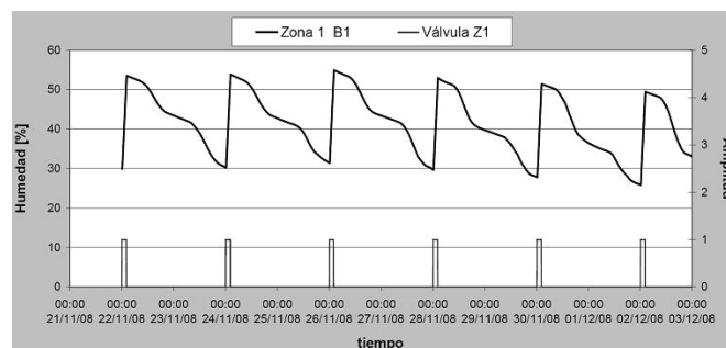
Figura 19. Ensayo N° 1. Controlador de riego operando en modo temporizado, con parámetros P=48hs y T=5hs.
