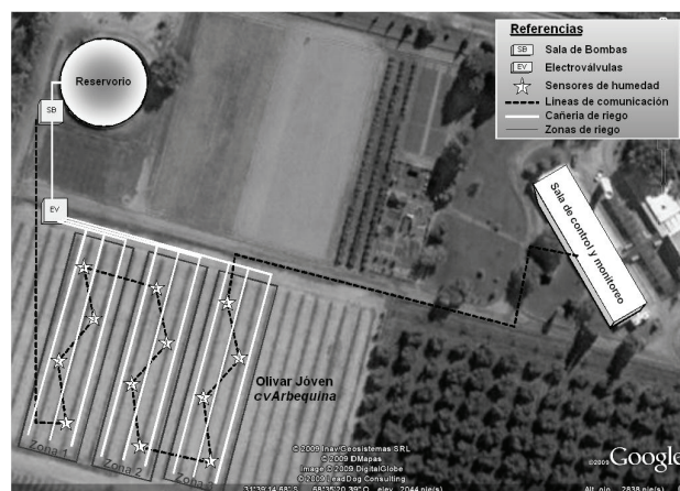
Figura 4. Fotografía aérea del lugar de experimentación y descripción gráfica de la planta piloto diseñada.
