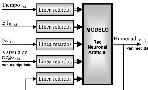
Figura 16: Modelo de simulación no-lineal de múltiples entrada y una salida (MISO).
