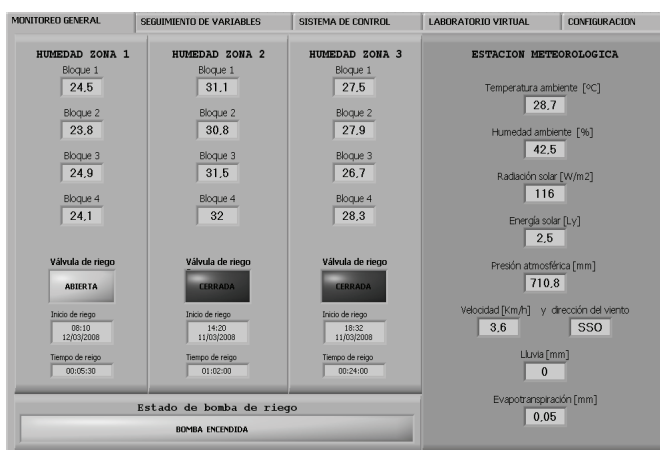
Figura 11. Pestaña de monitoreo general . Se presenta el estado actual de las variables medidas de la planta piloto.
