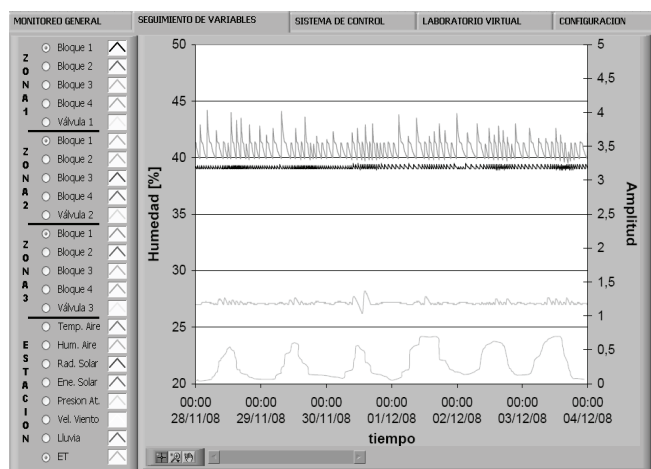
Figura 12. Pestaña de seguimiento de variables . Corresponde a la base de datos del sistema y se permite el seguimiento en forma gráfica de las variables medidas de la planta piloto.
