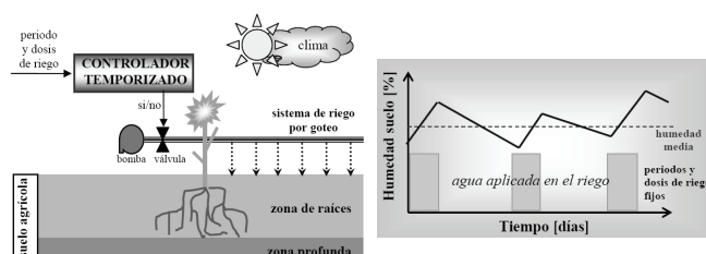
Figura 1. Sistema de riego temporizado (lazo abierto). Aplicación de dosis de riego fijas en periodos constantes.
