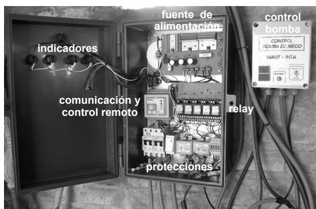
Figura 7. Componentes del tablero electrónico de control.
