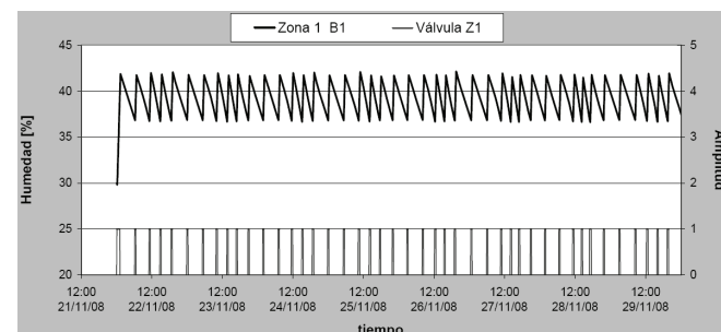
Figura 20. Ensayo N° 2. Controlador de riego operando en modo automático, con límite superior 40% y límite inferior 37% .
