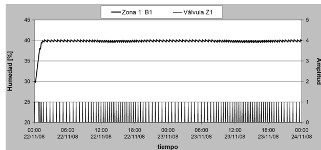
Figura 21. Ensayo N° 3. Controlador de riego operando en modo predictivo, humedad de referencia constante en 40%.
