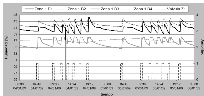
Figura 22. Experimento a campo N° 1. Controlador de riego configurado en modo automático , límite superior 41% y límite inferior 40%.
