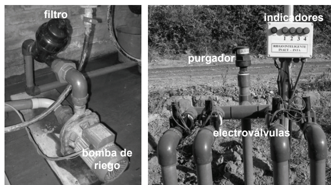
Figura 8: Elementos de distribución de agua del sistema de riego
