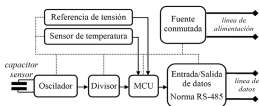
Figura 6. Esquema general del sensor de humedad utilizado en la planta piloto.
