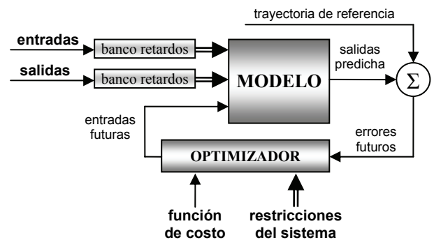
Figura 15: Estructura básica del CPBM.
