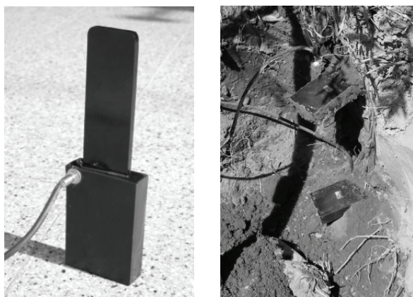
Figura 5. Sensor de humedad tipo capacitivo empleado a campo. Instalación del sensor en la zona de las raíces del olivo.
