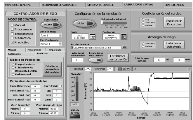
Figura 17. Pestaña de laboratorio virtual. Entorno de simulación y configuración del controlador de riego
