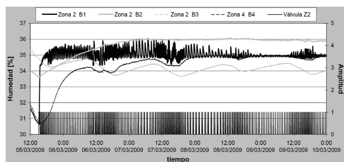
Figura 23. Experimento a campo N° 2. Controlador de riego configurado en modo predictivo , humedad de referencia constante en 35%.
