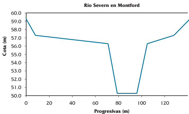
Figura 5. Sección transversal – río Severn en Montford
