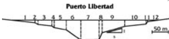
Figura 6. Secciones transversales – Alto río Paraná
