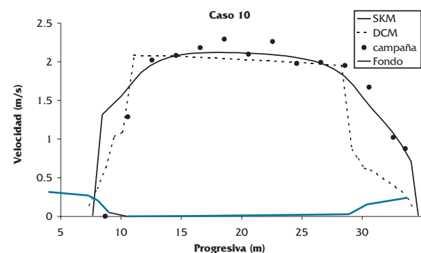
Figura 23. Resultados caso 10 – río La Suela
